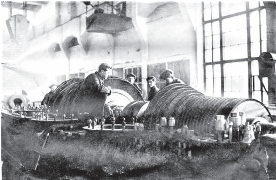
■ Установка ротора турбины – процесс, требующий мастерства и максимальной ответственности. Кемеровская ГРЭС, 1940-е годы.
