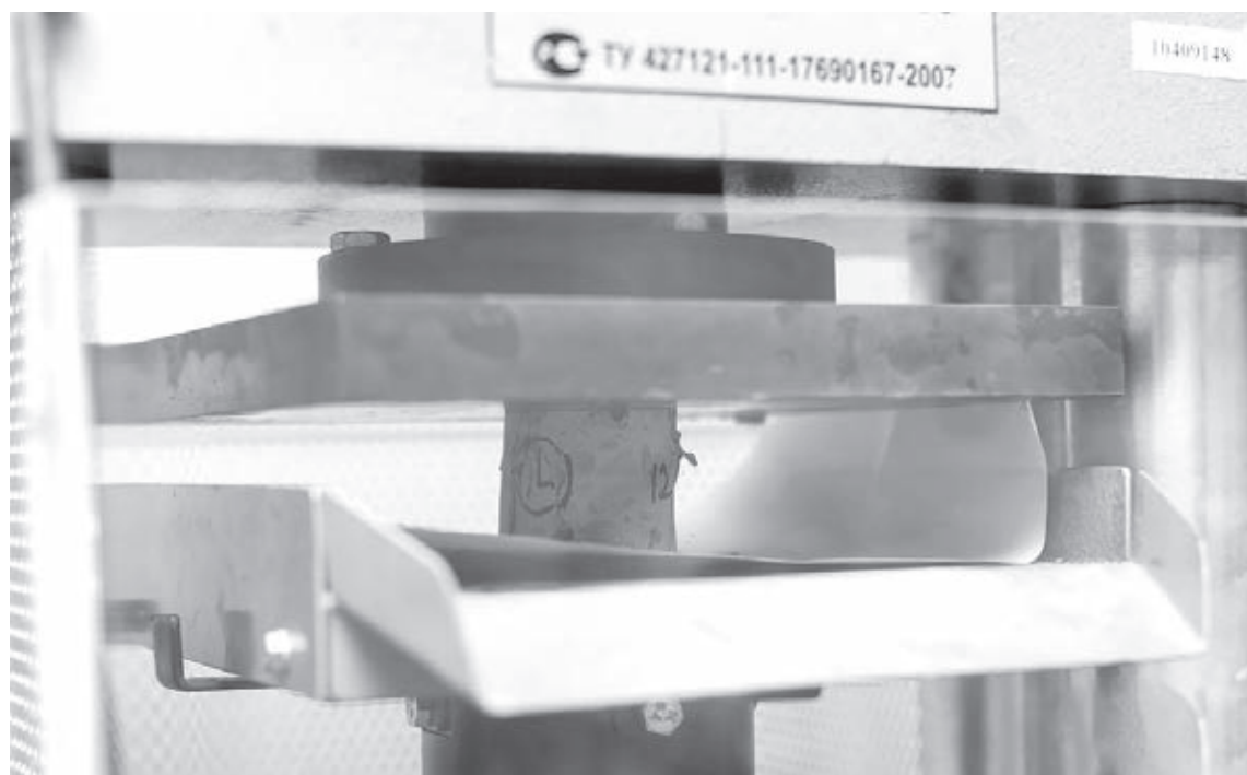
■ Испытания бетонной смеси с добавлением ЗШМ. Фото sibgenco.online.
