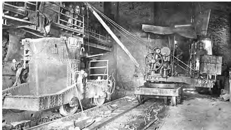
Разливочный пролет мартеновского цеха 1945-1946 гг.
