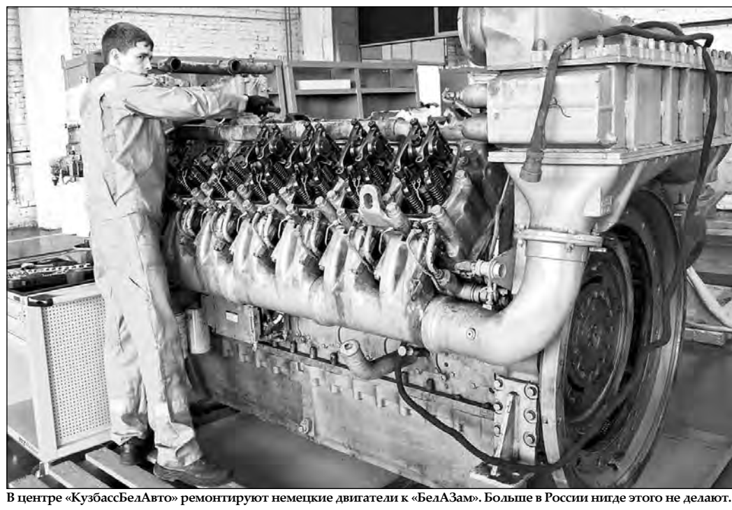
В центре «КузбассБелАвто» ремонтируют немецкие двигатели к «БелАЗам». Больше в России нигде этого не делают.
